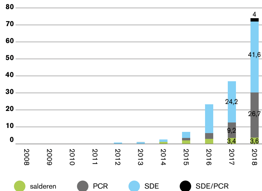
Zon: totaal collectief vermogen naar type regeling in MWP
