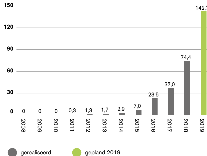
Zon: ontwikkeling totaal collectief vermogen in MWP
